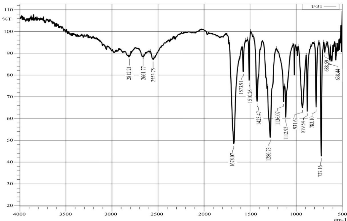
Fig. 6 Terephthalic acid IR spectrum
